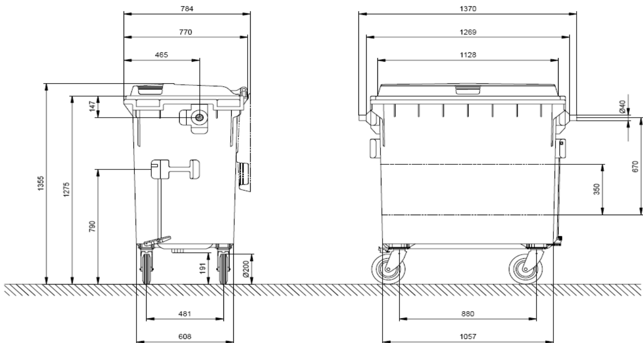
Dibujo acotado (medidas en mm.)
